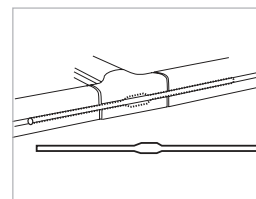
I-spojka pro zpevnění tříramenné koncovky 3204
